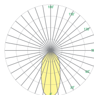
MED 48° Beam
